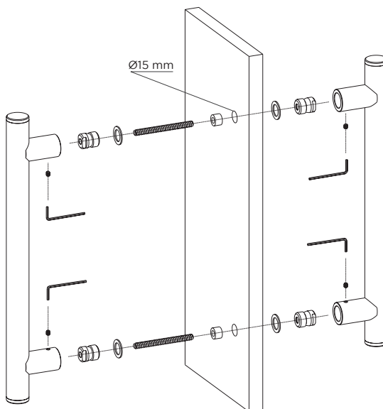
MONTAŻ POCHWYTU DWUSTRONNEGO DO DRZWI SZKLANYCH
