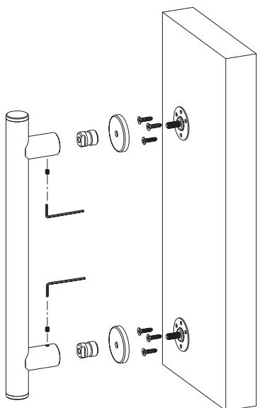
MONTAŻ POCHWYTU JEDNOSTRONNEGO PRZY UŻYCIU ROZETY STABILIZUJĄCEJ
