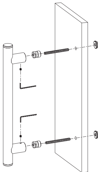
MONTAŻ POCHWYTU JEDNOSTRONNEGO NA PRZESTRZAŁ
