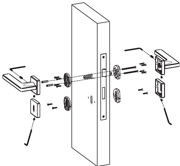
MONTAŻ KLAMKI NA ROZECIE
