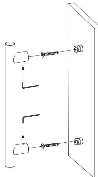
MONTAŻ POCHWYTU JEDNOSTRONNEGO NA DREWNOWKRĘT
